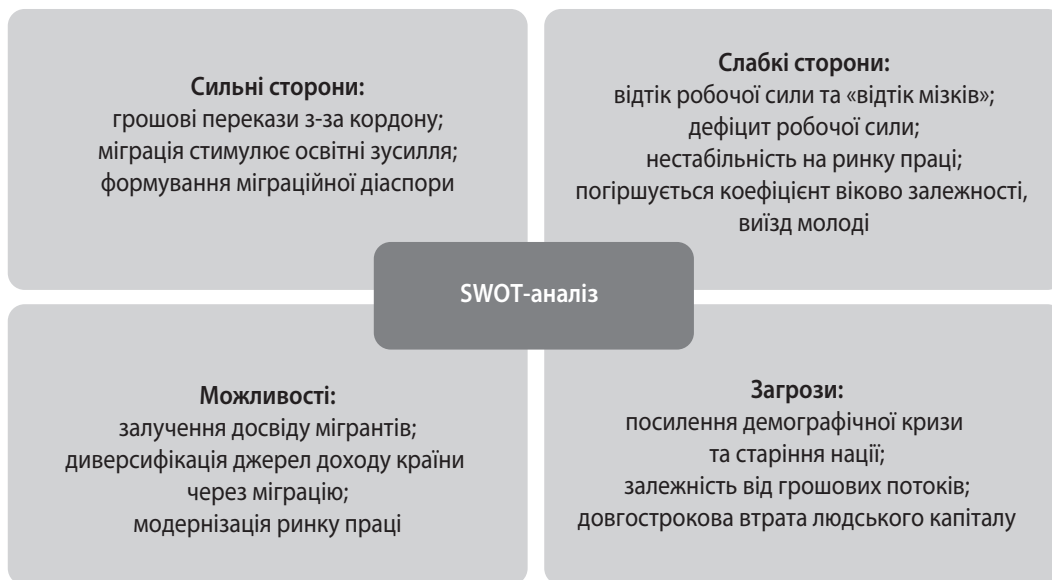
Рис. 3. SWOT-аналіз міждержавної міграції України
